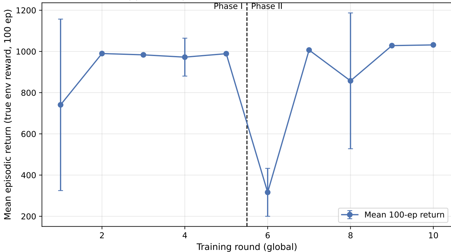
Hopper-v4: episodic return per round (Phase I \rightarrow II)
