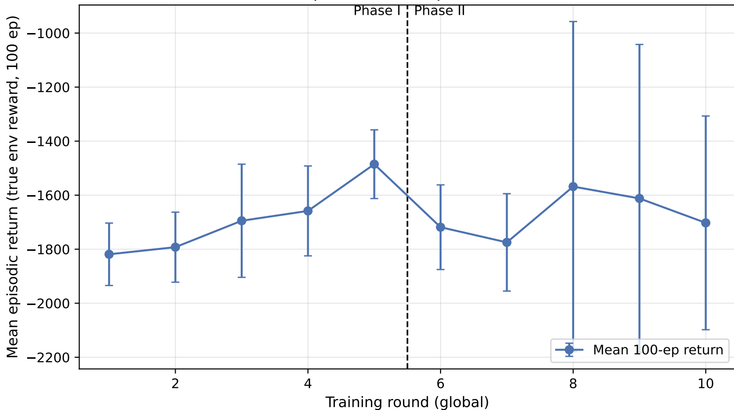
Pendulum-v1: episodic return per round (Phase I → II)
