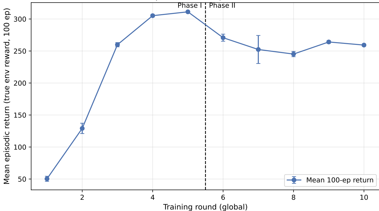
Swimmer-v4: episodic return per round (Phase I → II)
