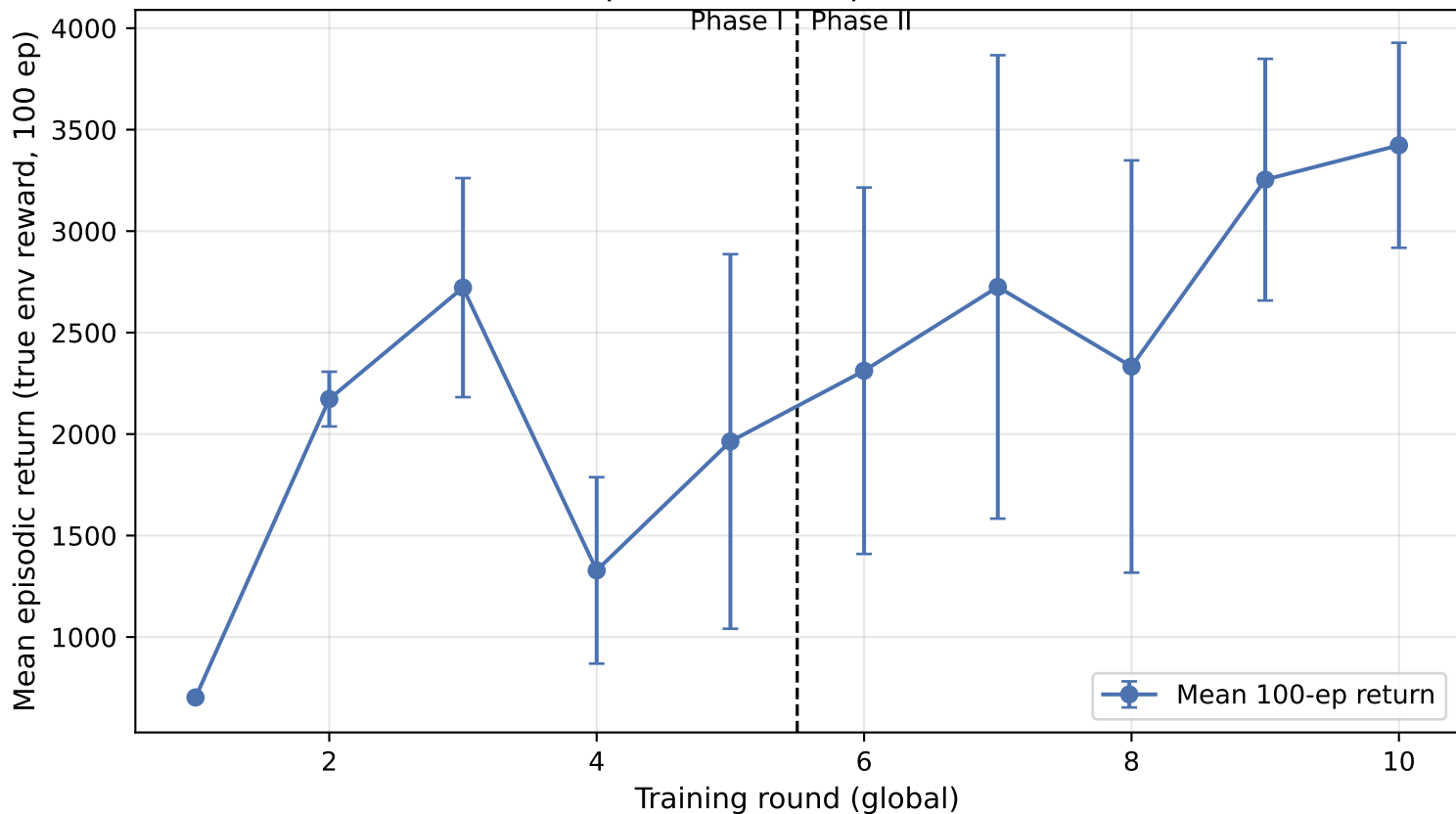
Walker2d-v4: episodic return per round (Phase I \rightarrow II)
