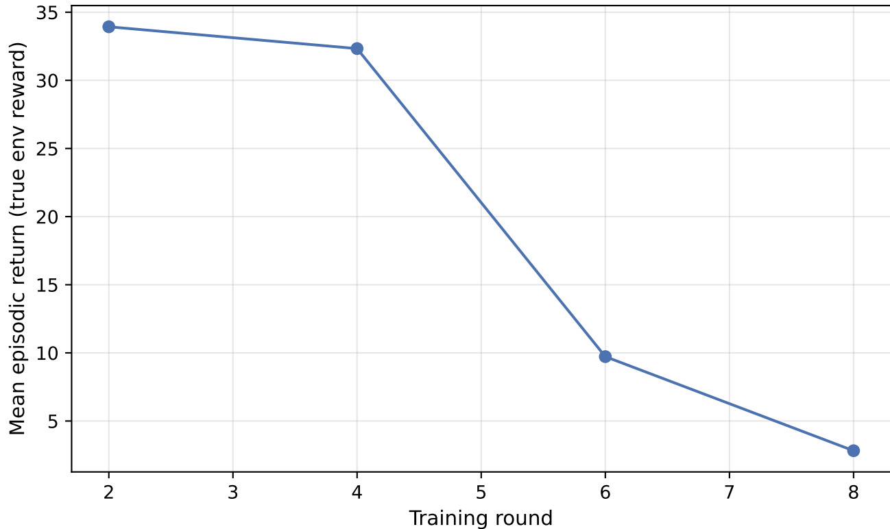
Swimmer-v4: episodic return per round
