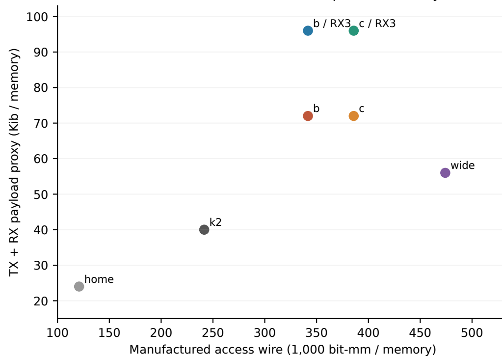
(d) RX3 costs another 24 Kib per k3 memory
