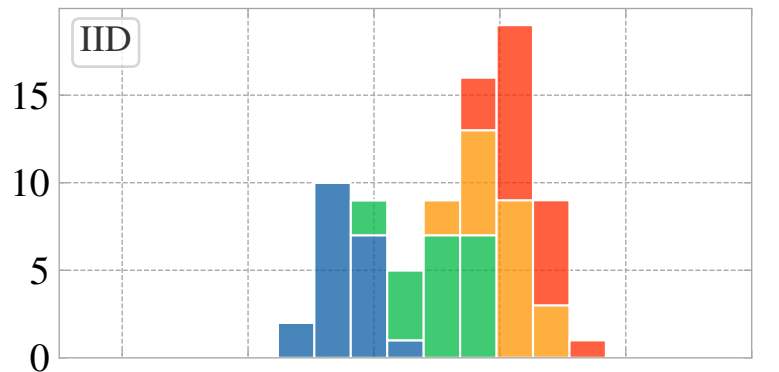
HeteroFL
