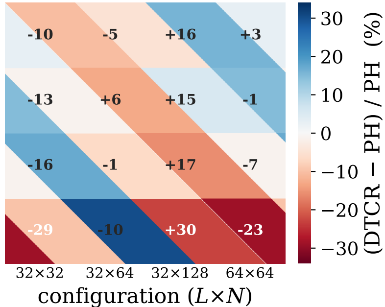
GTX 1070 (Pascal)
