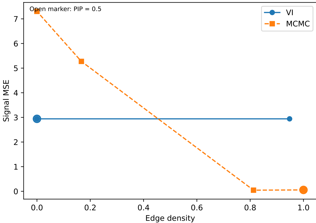
embed_output: edge_group
