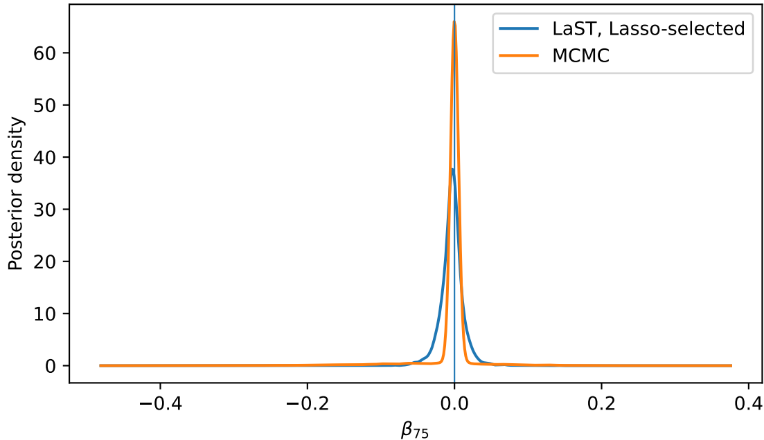
True-zero marginal posterior recovery seed 400, beta_75
