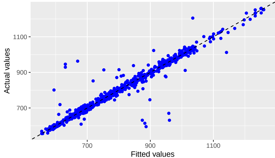
Actual vs. Fitted Values: Drift Model
