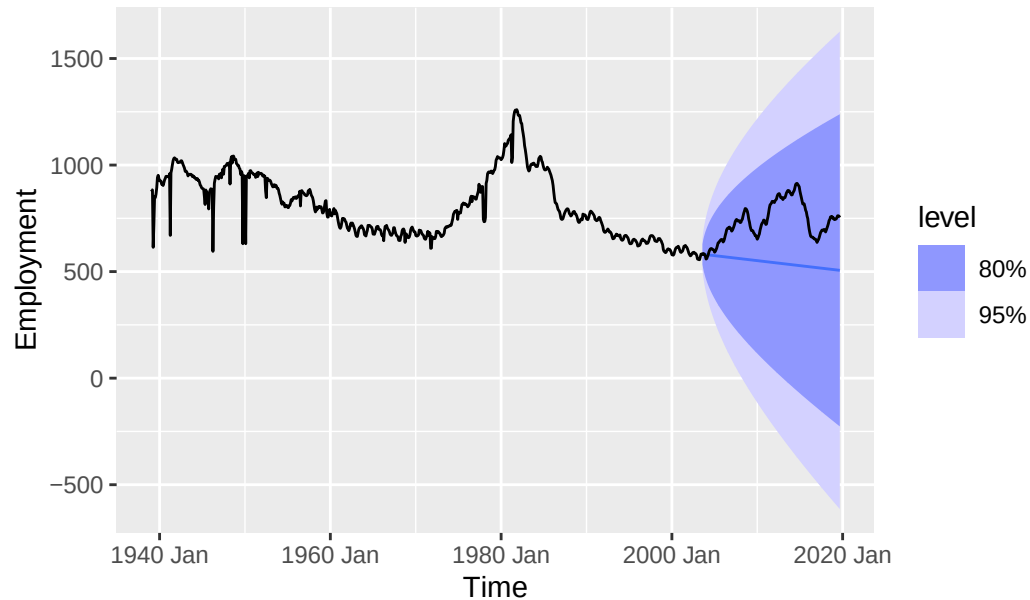
Actual vs. Forecast: Drift Model
