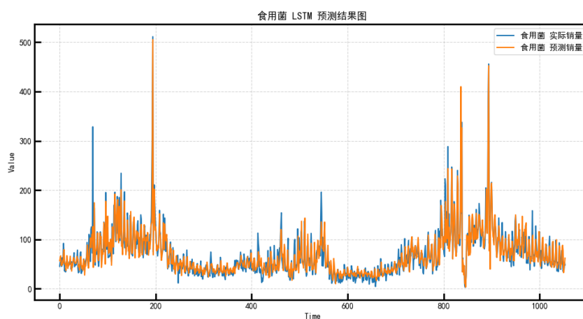
图 26 食用菌 LSTM
