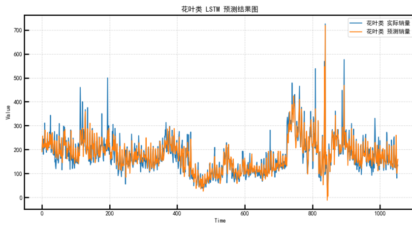
图 21 花叶类 LSTM
