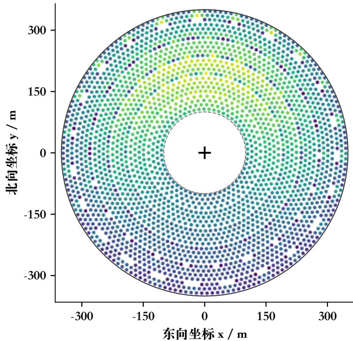
(a) 统一镜型：2425 面
