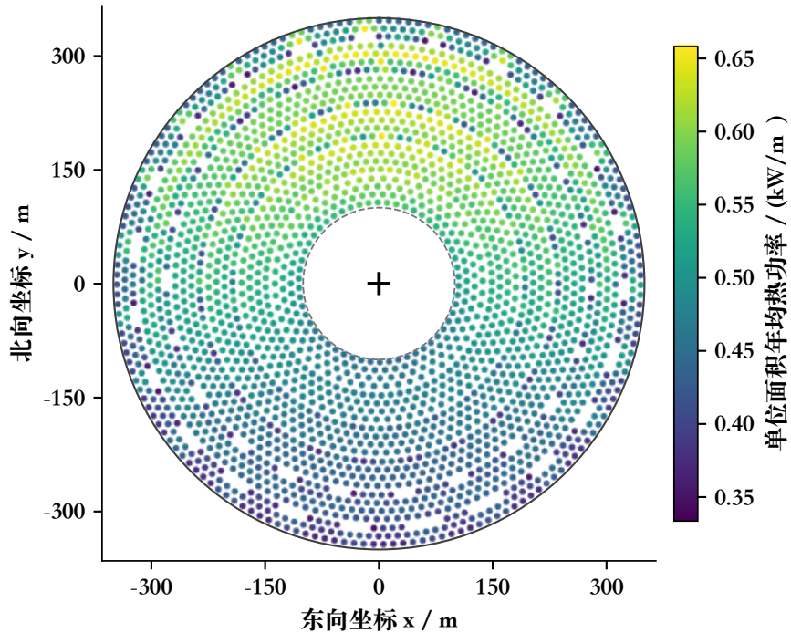
(b) 异构镜型：2404 面
