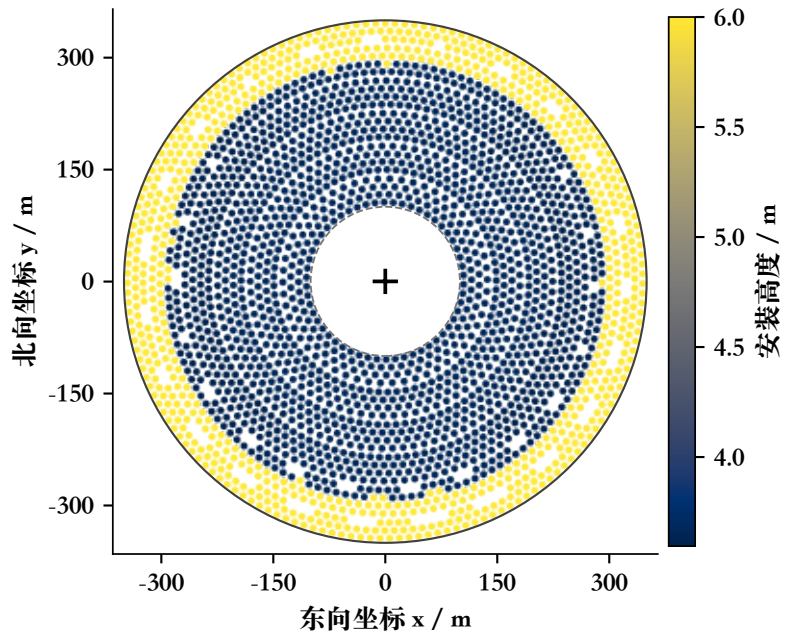
(b) 安装高度分布
