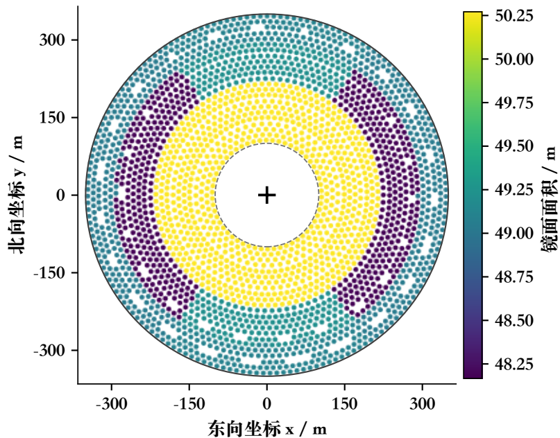
(a) 镜面面积分布
