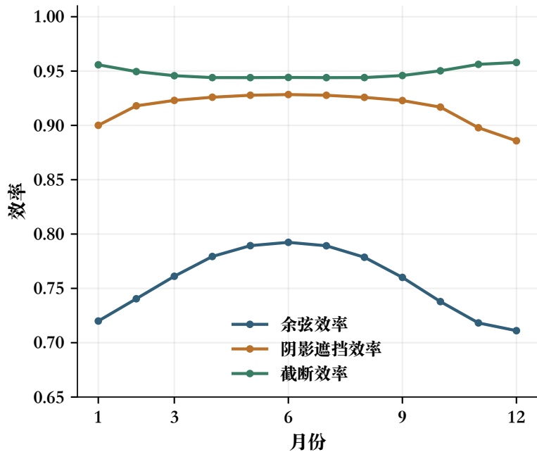
(b) 逐月平均分项效率
