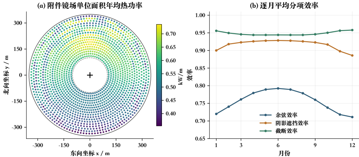
图 2 给定镜场的空间产热差异及逐月光学效率
