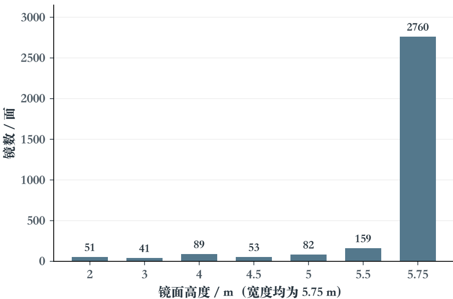
(a) 第三问镜面规格分布
