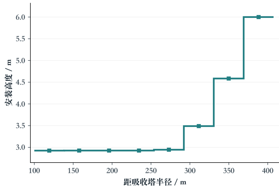
(b) 八个径向区间的安装高度
