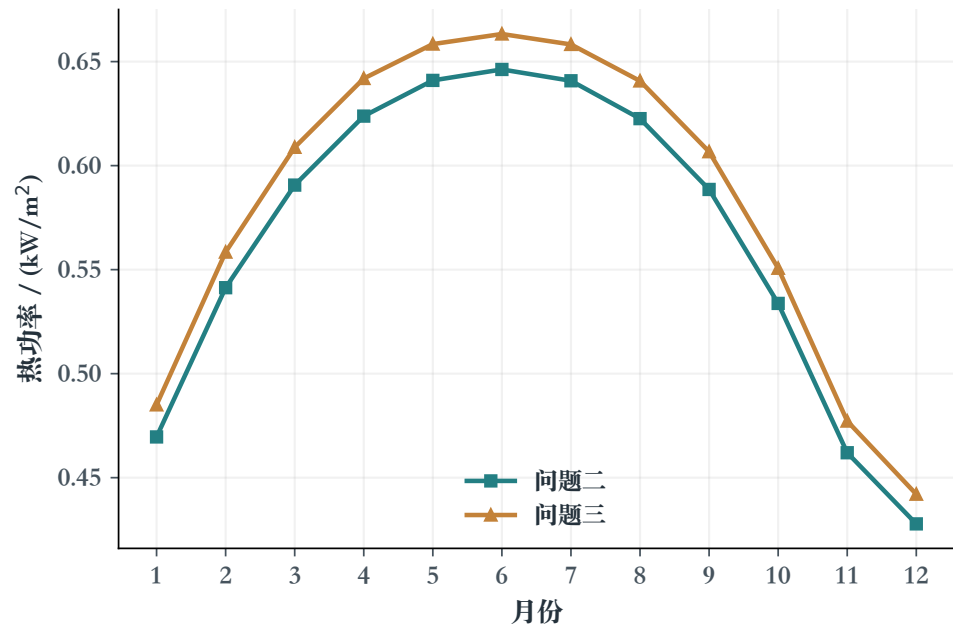
(b) 第二、三问单位面积热功率
