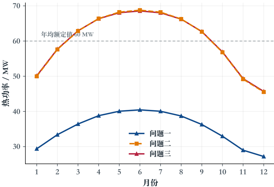
(a) 三问逐月平均热功率
