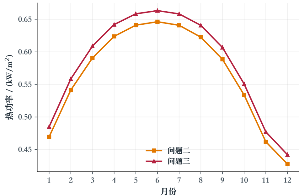
(b) 第二、三问单位面积热功率
