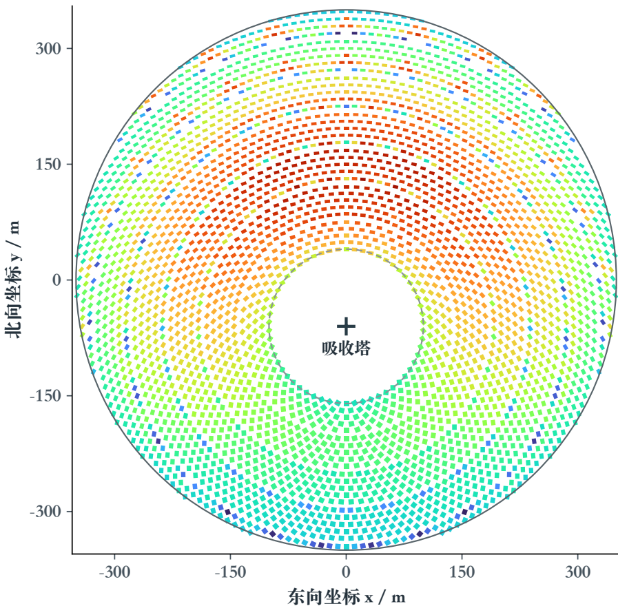
(a) 问题二: 3,219 面
