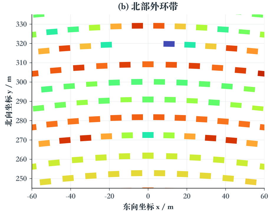
第三问局部放大：镜面使用真实尺寸与参考时刻投影，可见交错环距和不同矩形尺寸。
