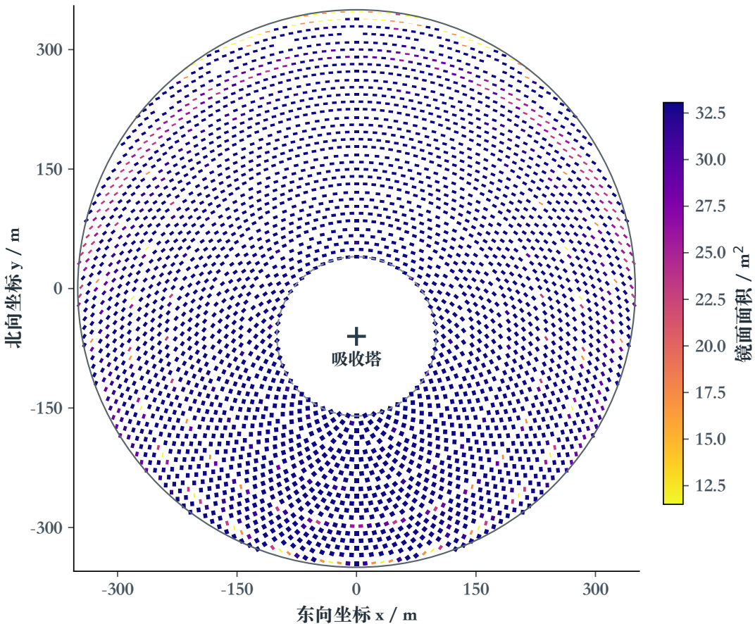
(a) 镜面面积
