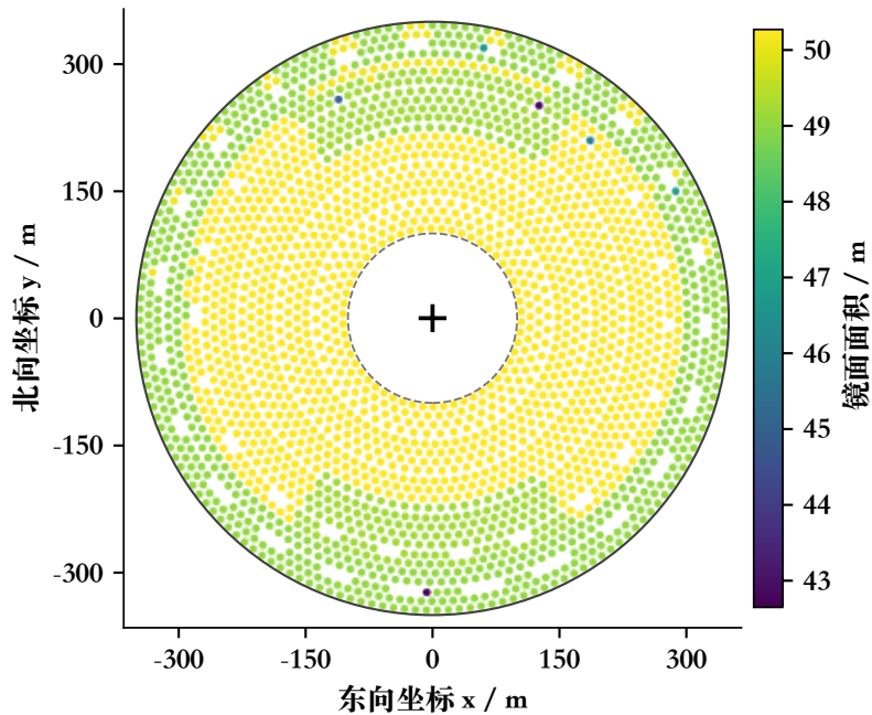
(a) 镜面面积分布
