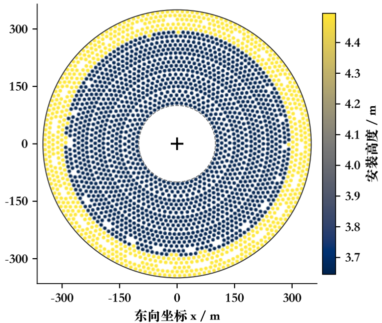
(b) 安装高度分布
