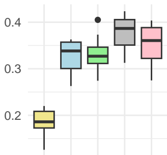
MAP@100
