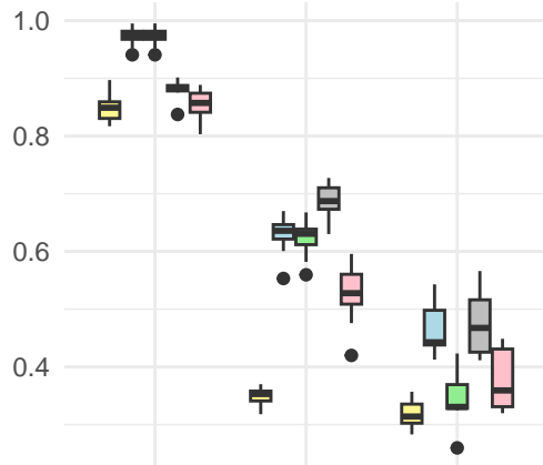
Prec@5
