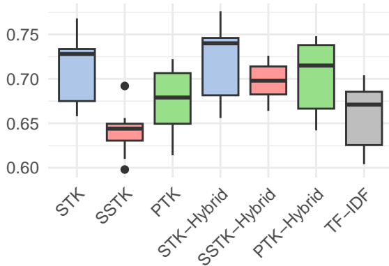
Prec@5
