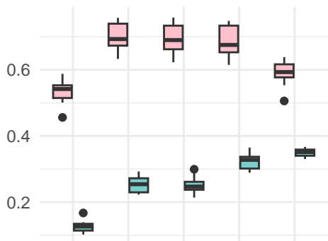
MAP@100
