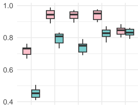
Prec@5
