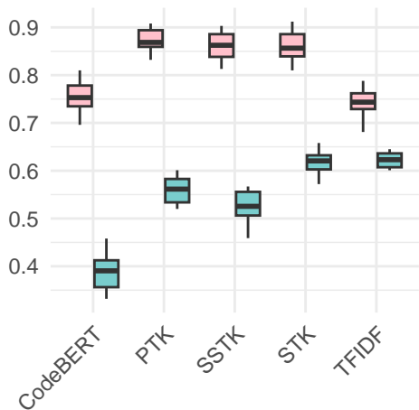
Prec@10
