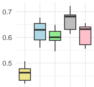
Prec@10
