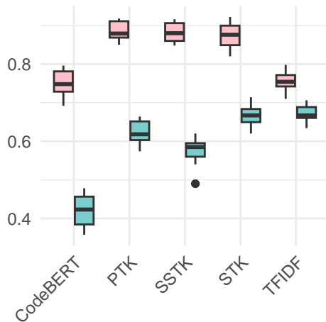
Prec@5
