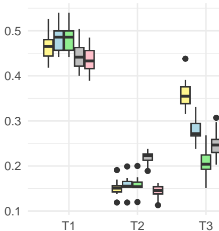
Prec@10
