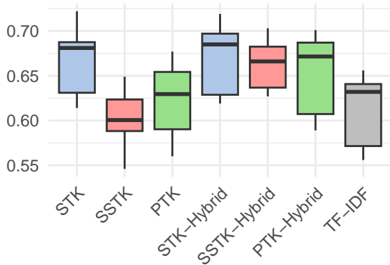
Prec@10
