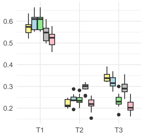
Prec@5
