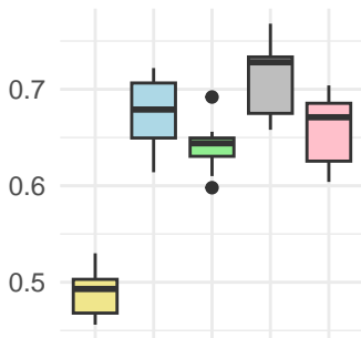
Prec@5
