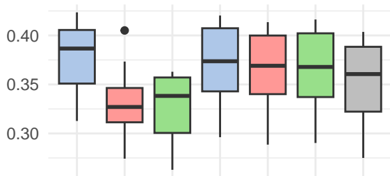
MAP@100
