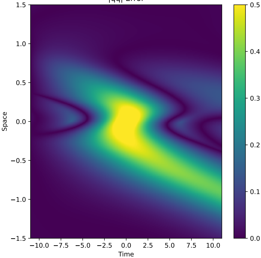
|qq| Error
