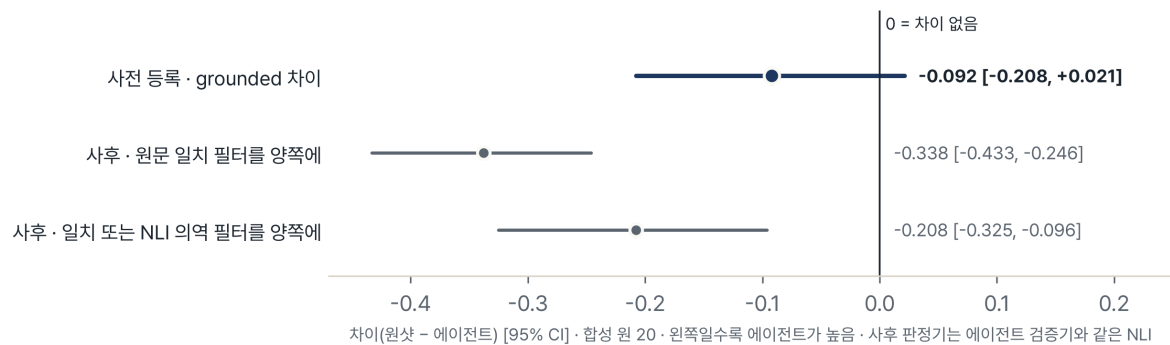
그림 4. 원샷 대비 차이와 95% CI. 사전 등록 판정(강조)은 CI가 0을 포함해 차이 확인 안 됨이다. 아래 두 줄은 사후 분석이고 판정기가 에이전트 검증기와 같은 NLI라 에이전트에 유리하다. 값은 docs/numbers.md 1-5절
