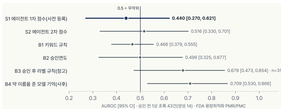
그림 3. 후향 검증 AUROC와 95% CI. 사전 등록 1차 점수 S1(강조)의 CI가 0.5(무작위)를 포함한다. 값은 docs/numbers.md 1-4절
