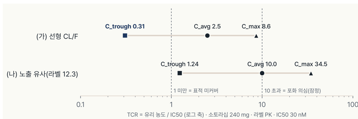
그림 1. 소토라십 240 mg의 TCR. 같은 용량에서도 지표와 PK 가정에 따라 미커버(1 미만)부터 포화 의심(10 초과, 잠정)까지 갈린다. 값은 evidence/tcr_240mg.json
