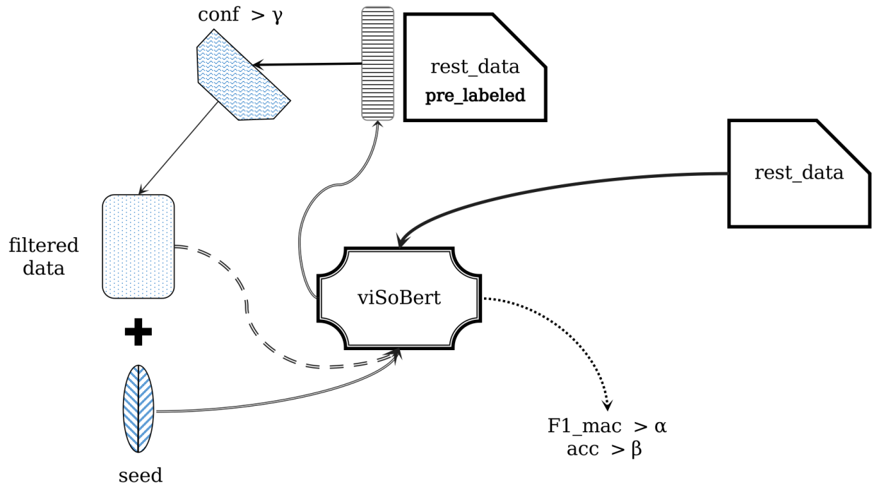
Figure 1: Quy trình gán nhãn tự động
