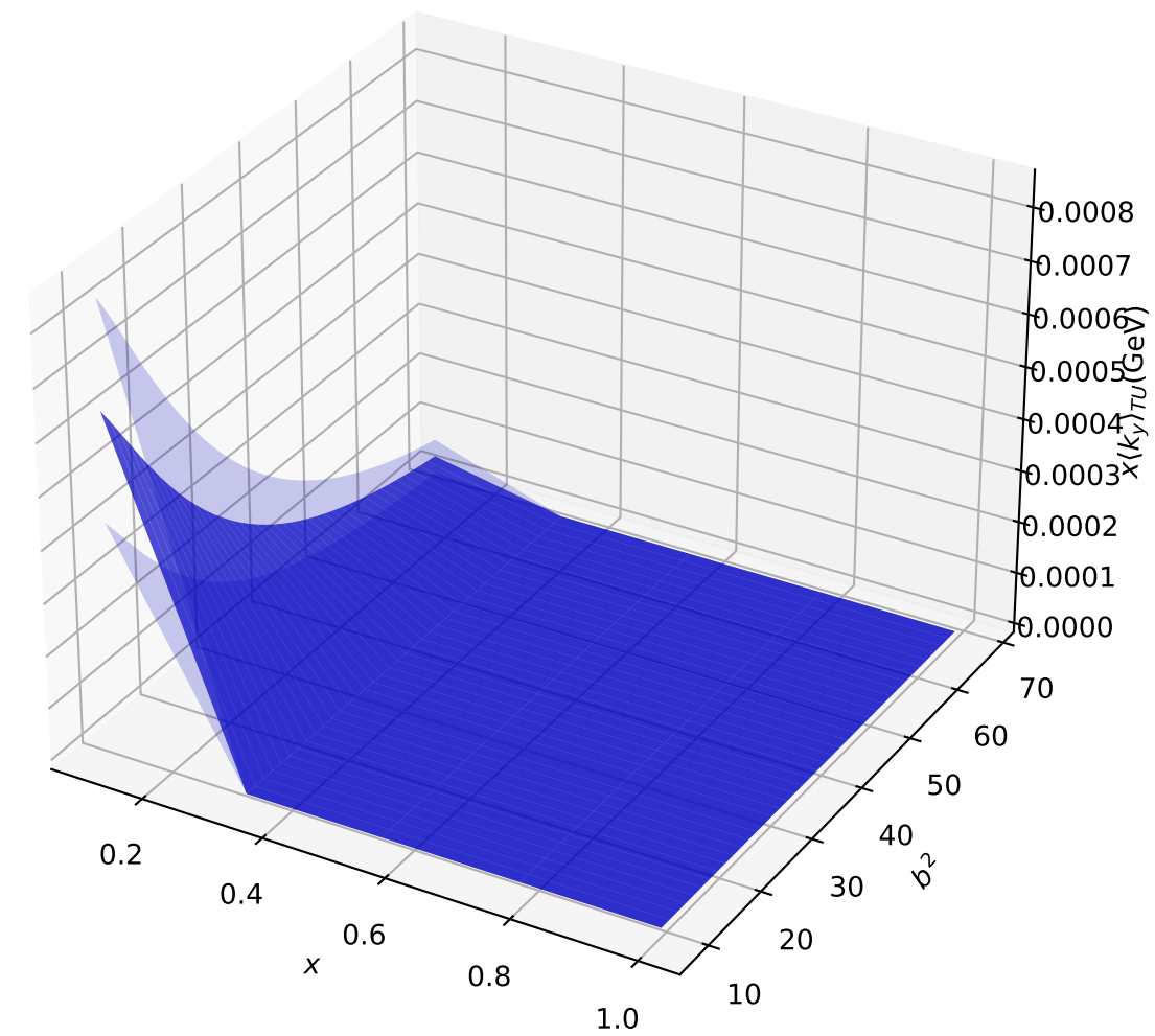
x\langle k_y \rangle_{TU}(\text{GeV}) (P_L=25)
