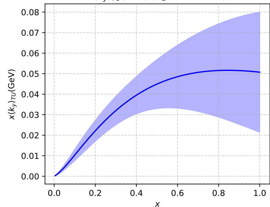
x\langle k_y \rangle_{TU}(\text{GeV}) (P_L=-4, b^2=36)
