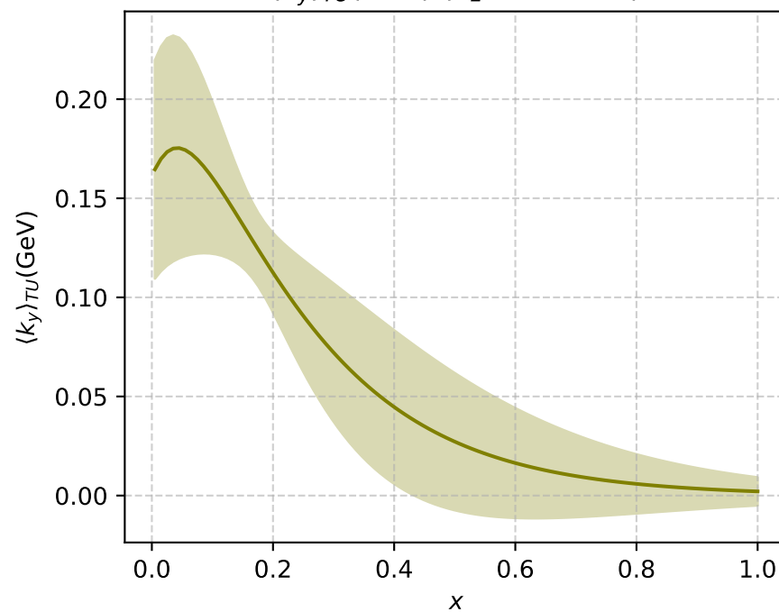
\langle k_y \rangle_{TU}(\text{GeV}) (P_L=-4, b^2=9)
