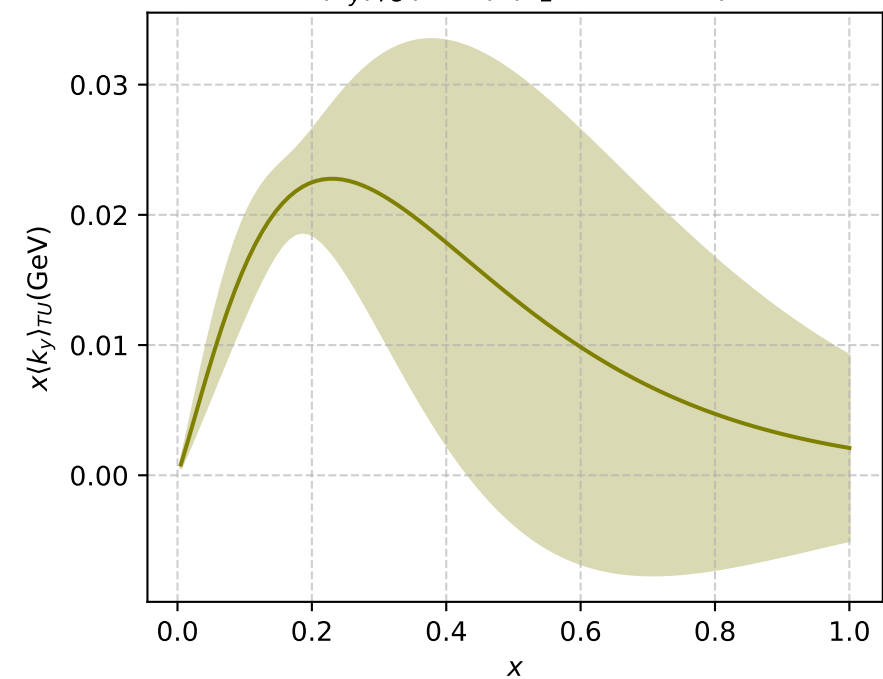
x\langle k_y \rangle_{TU}(\text{GeV}) (P_L=-4, b^2=9)
