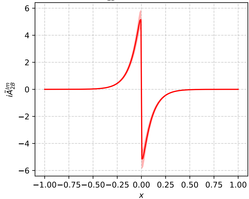
i\tilde{A}_{2B}^{Im} (P_L=-3, b^2=9)
