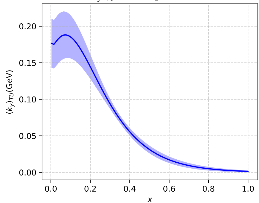
\langle k_y \rangle_{TU}(\text{GeV}) (P_L=-3, b^2=9)
