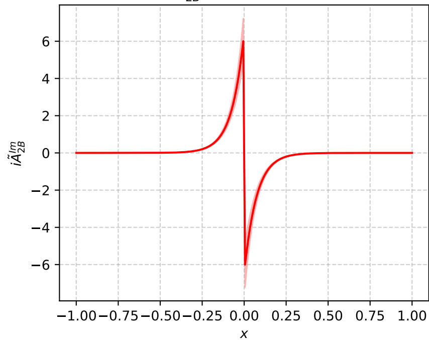
i\tilde{A}_{2B}^{Im} (P_L=-4, b^2=9)
