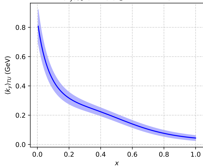
\langle k_y \rangle_{TU} \text{ (GeV)} (P_L=-1, b^2=50)
