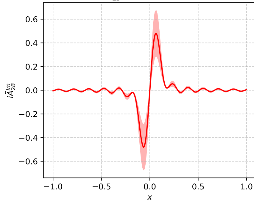
i\tilde{A}_{2B}^{Im} (P_L=-4, b^2=36)
