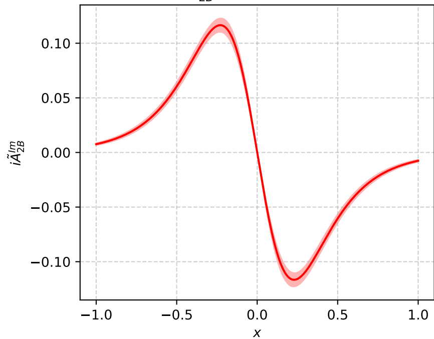
i\tilde{A}_{2B}^{Im} (P_L=-1, b^2=9)
