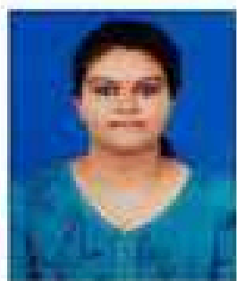
Kirubah M (8.51)
