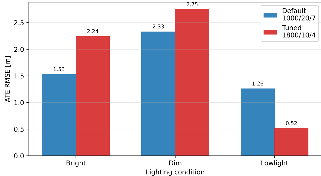
ORB-SLAM3 parameter ablation, t03
