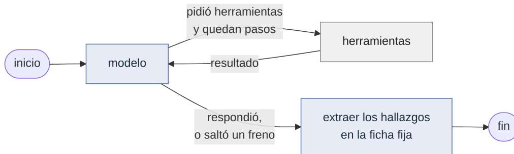
Figura 2. El bucle de un agente. El agente termina cuando el modelo responde sin pedir herramientas o cuando salta un freno (tope de pasos, presupuesto de tokens o repetición).
