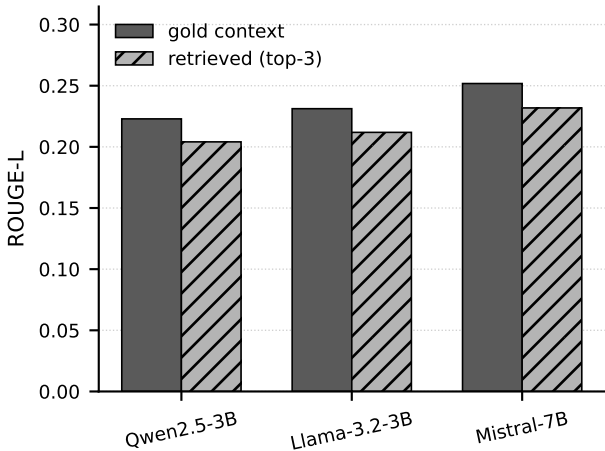
Retrieval-attributable gap
