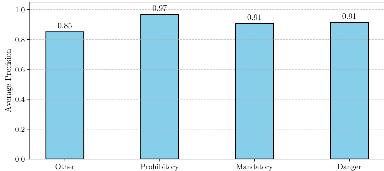
Average Precision per Class
