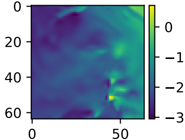
HR data
