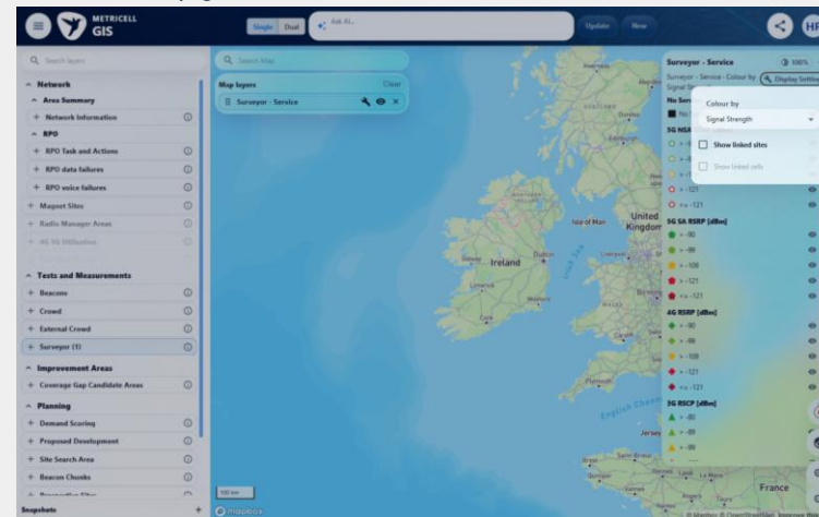
E16 - criterion-3-after-close.png
