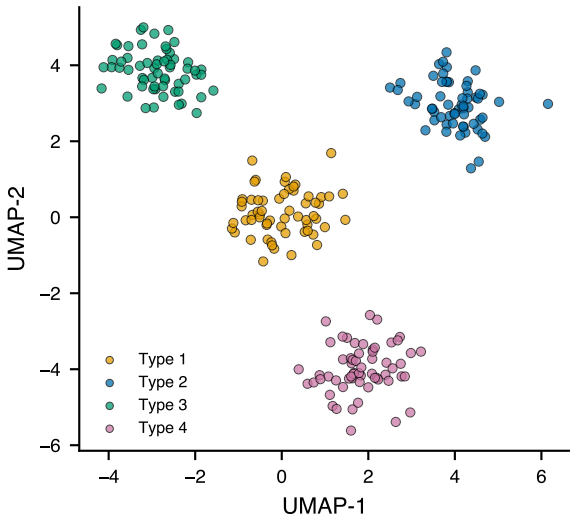
Embedding (UMAP-style)
