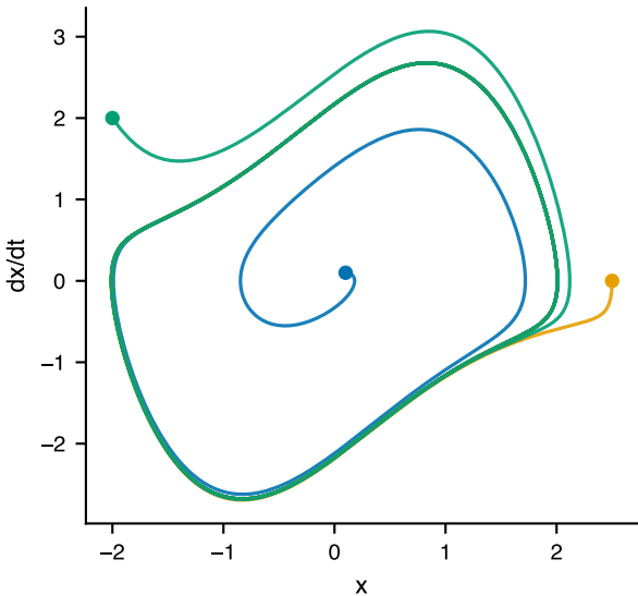
Phase portrait (Van der Pol)
