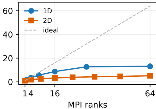
roadNet-PA
