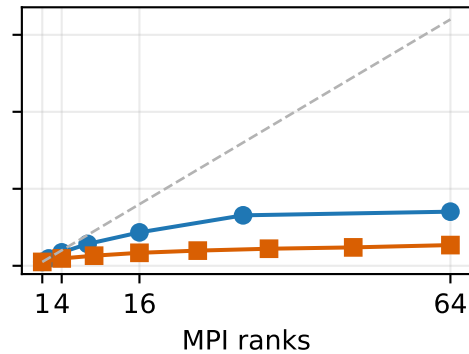
roadNet-TX
