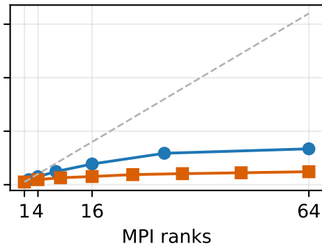
roadNet-CA
