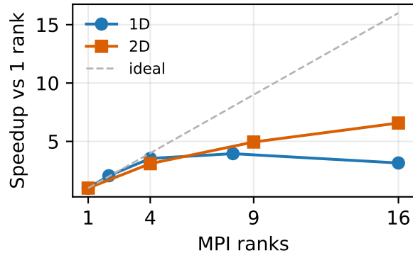
large_dense
