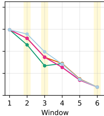
K = 200
