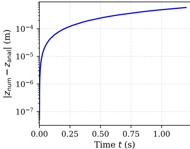
(b) Numerical error
