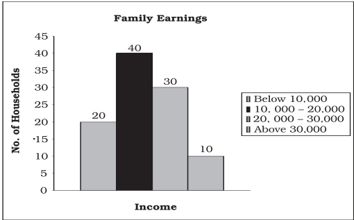
Fig. 8.3: Histogram
